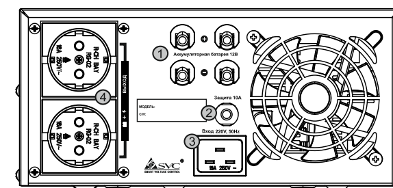
DIL-1200
